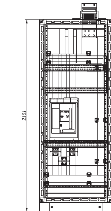
Вид спереди
