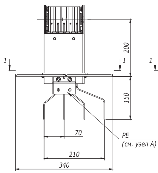
3P+N+PE
