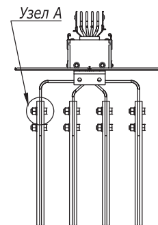
Узел А
