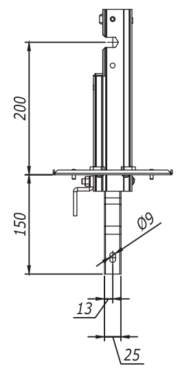
Узел А Заземляющий контакт
