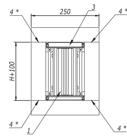
Огнестойкий проход через стену. Вид спереди
