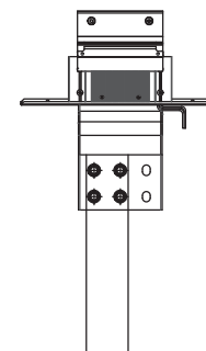
Фрагмент открытой части присоединительной секции шинопровода
