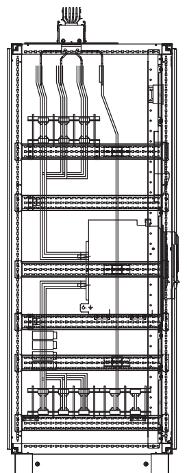
Вид сбоку
