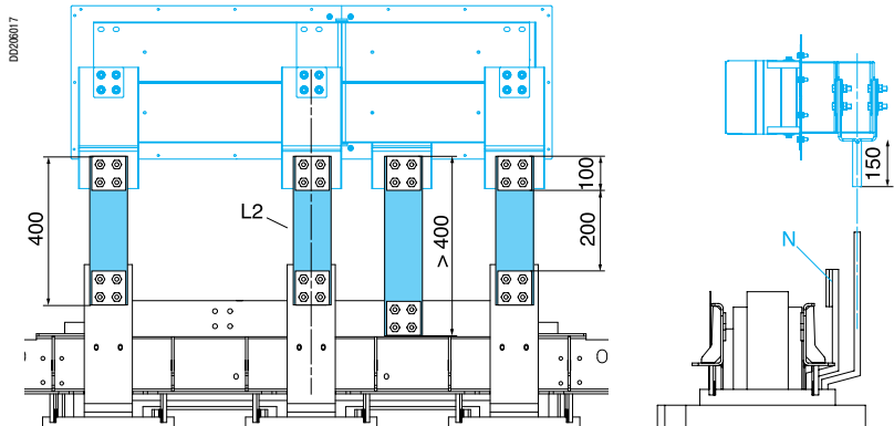
Универсальный блок TS7, установка «на ребро»
