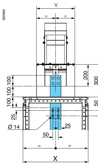
Вертикальный ввод
