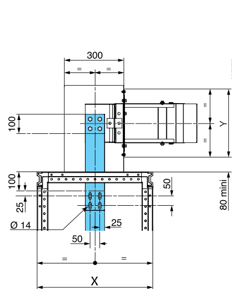
Горизонтальный ввод
