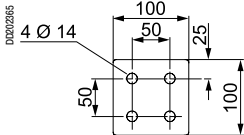
Медная пластина
