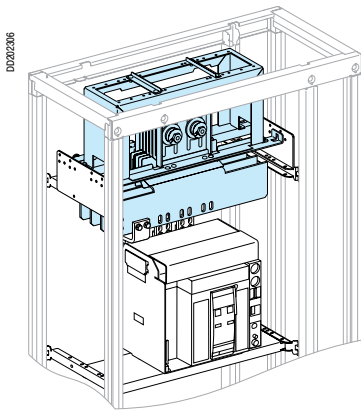
Щит Prisma
