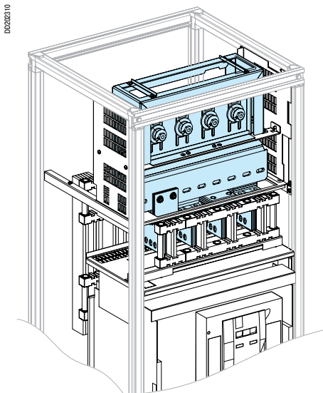
Щит Okken
