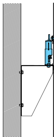
Крепление на настенном кронштейне
