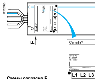
Схемы согласно F
