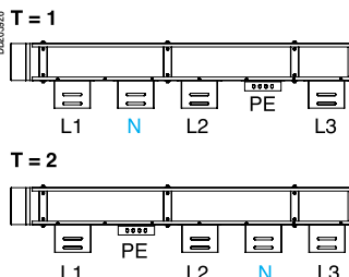
Схемы согласно F
