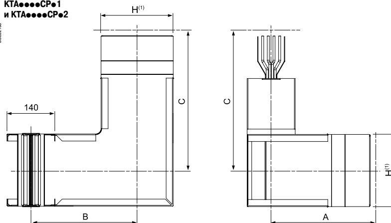
КТА...СР•3 и КТА...СР•4
