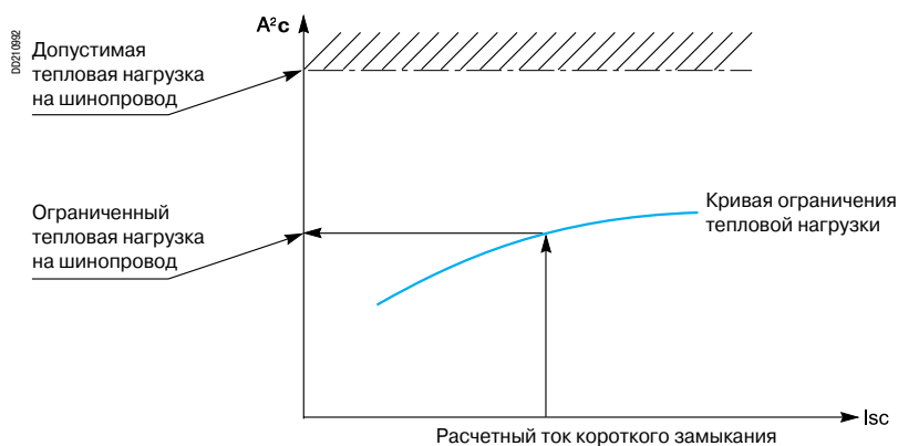
Проверка стойкости шинпровода к тепловой нагрузке
