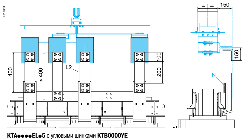
Универсальный блок TS7, установка «плашмя» с угловыми шинками
