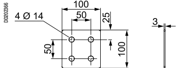
Оцинкованная стальная пластина
