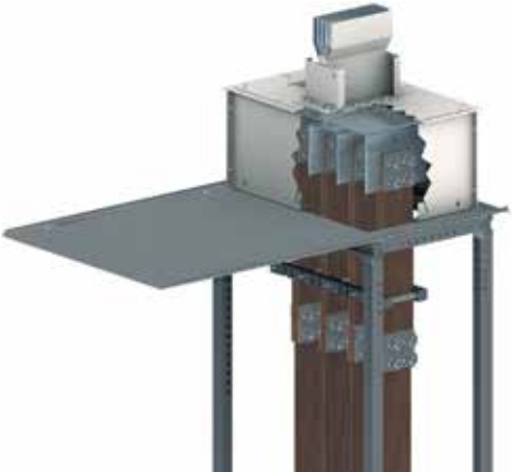
Универсальный вводной блок (рекомендованное расстояние между центрами - 115 мм)
