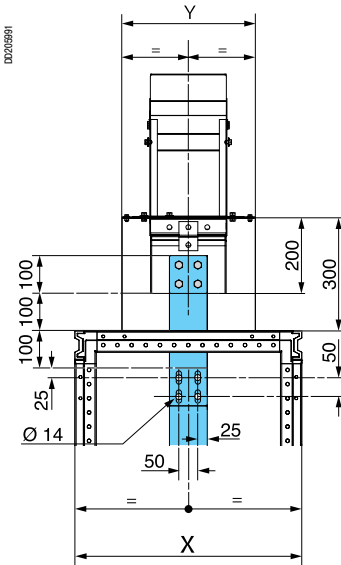
Вертикальный ввод
