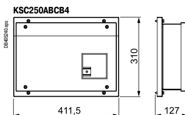
KSC250ABCB4
