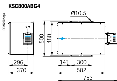
KSC800ABG4
