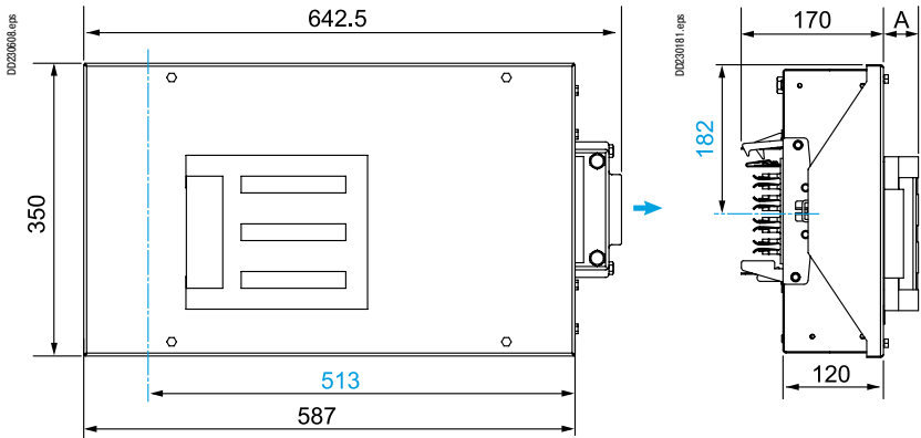
KSB●●HD502
