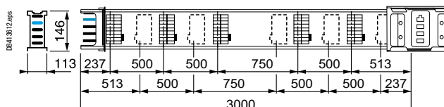
KSC●●●ED43010
