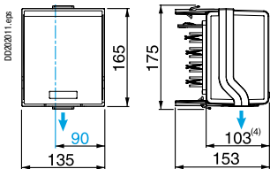
KSB32CF5
