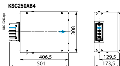
KSC250AB4
