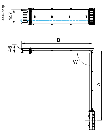
KSC...DLC4A 400 А
