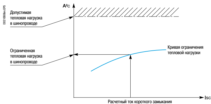
Ограничивающие свойства защиты BTS относительно тепловой перегрузки
