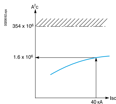
Ограничение энергии
