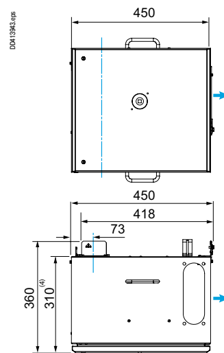
KSB250DD412
