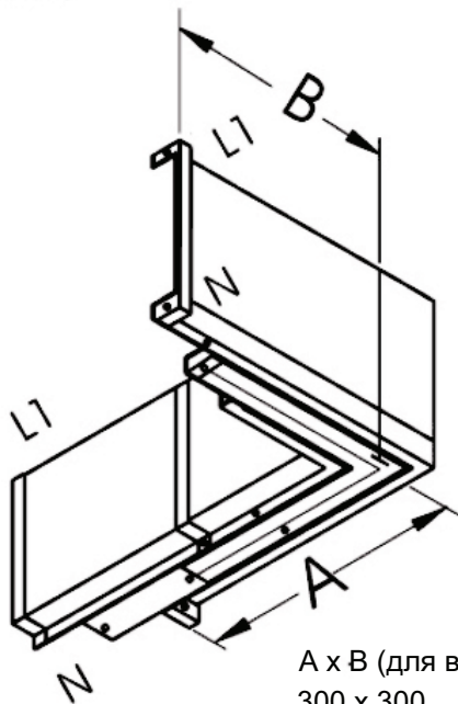
вертикальная секция угловая с поворотом шин по плоскости, исполнение - 1
