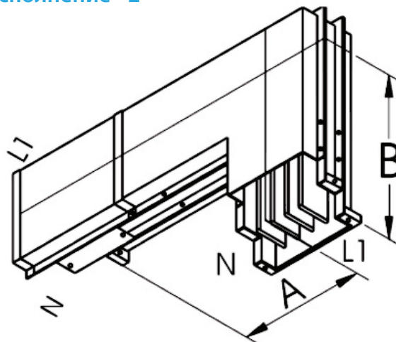
горизонтальная секция угловая с поворотом шин по ребру, исполнение - 2
