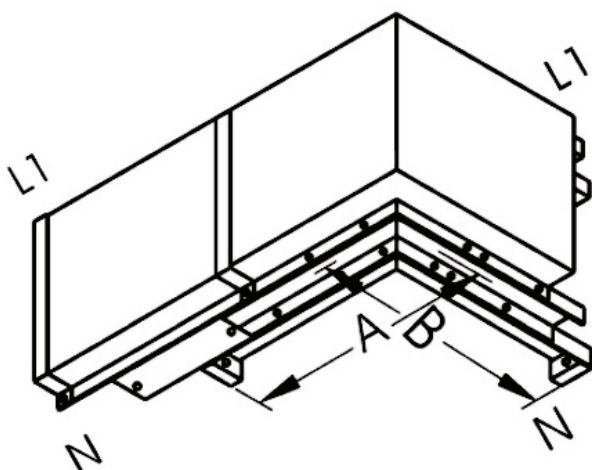
вертикальная секция угловая с поворотом шин по плоскости, исполнение - 2
