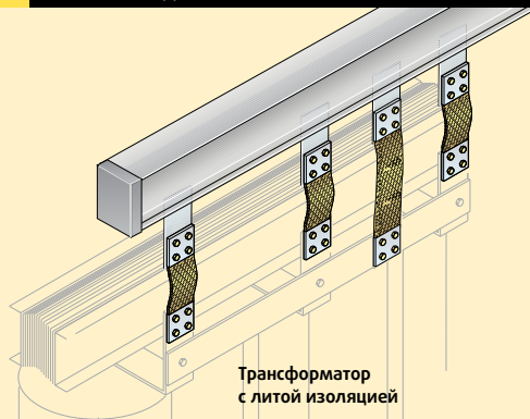
Сторона НН
