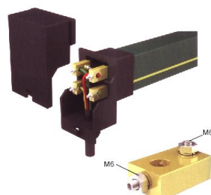
Подвод в разборе
