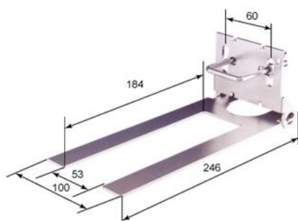
Кронштейн 1
