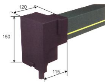
Концевой подвод
