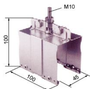
Подвес
