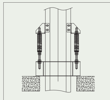
[Side View] / Вид сбоку
