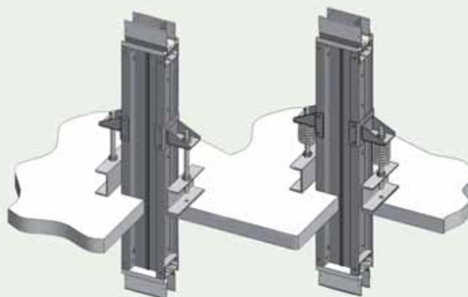
[RigidHanger] / Жесткая подвеска
