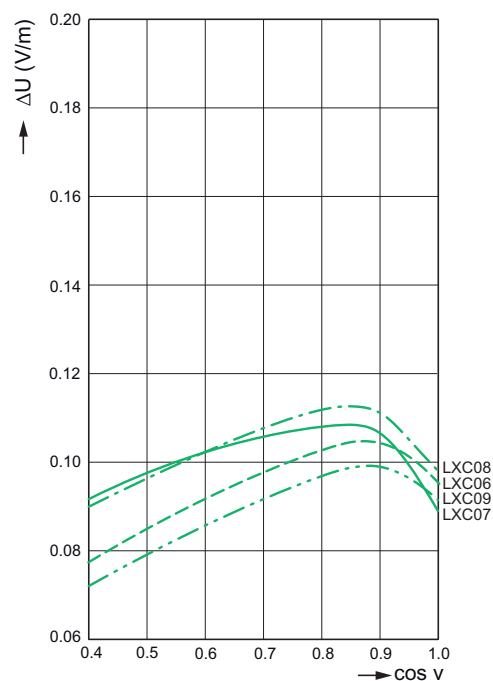
Падение напряжения LXC
