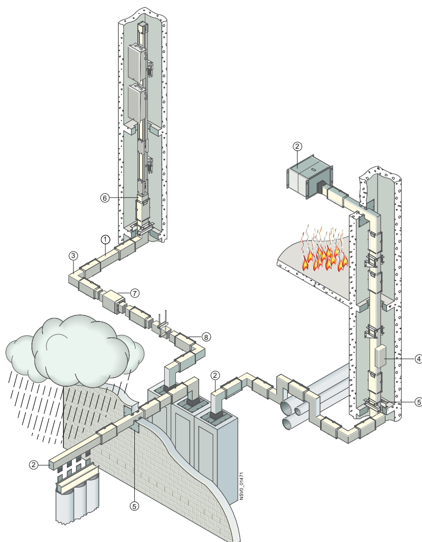
Рисунок 6-1 Система шинопровода LRC
