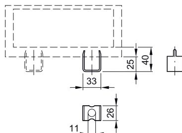
Рисунок 3-74 BD2-DSB
