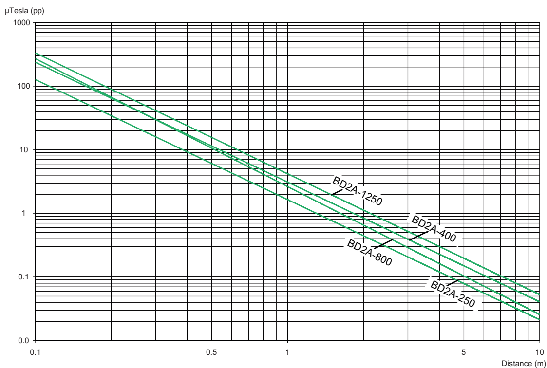
Рисунок 7-10 BD2 магнитные поля для систем Al 250 A, 400 A, 800 A, Cu 1250 A
