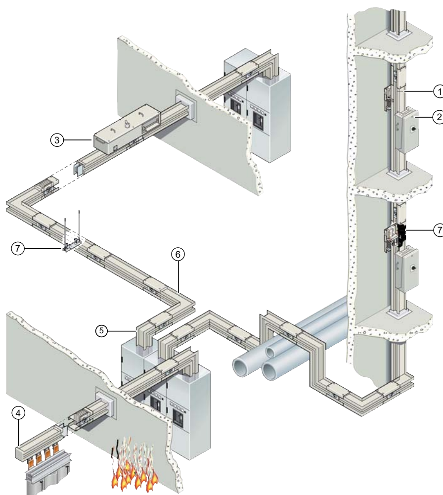
Рисунок 5-1 Обзор систем шинопровода LXA/LXC
