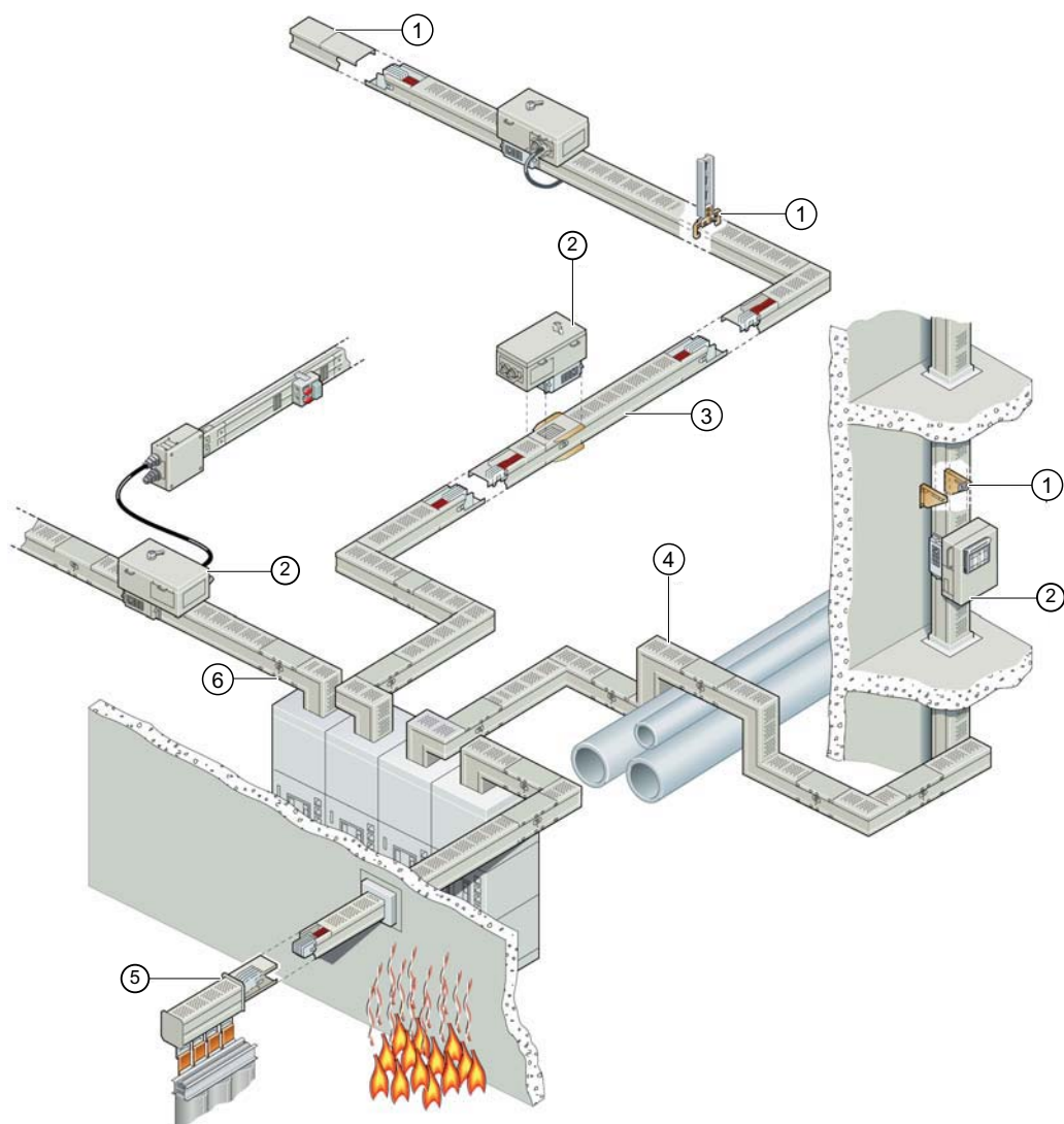
Рисунок 4-1 Обзор систем шинопровода LDA/LDC
