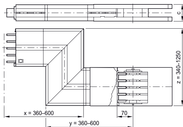
Рисунок 3-23 BD2-...-ZR-..., BD2-...-ZL-...
