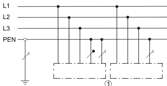
Рисунок 7-2 TN-C система
