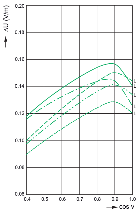
Падение напряжения LXC
