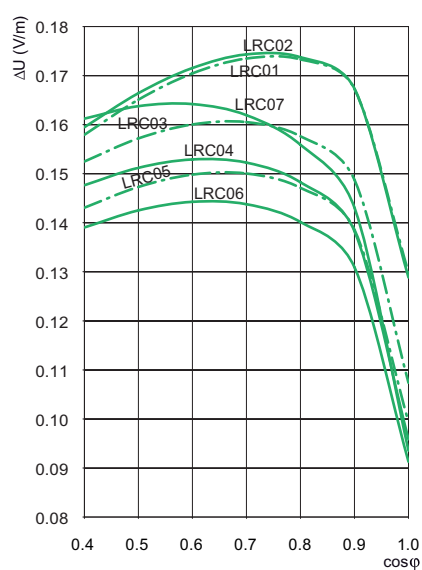
Падение напряжения LRC01 до LRC07
