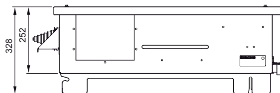
Рисунок 3-67 BD2-AK05/SNH2, BD2-AK06/SNH3
