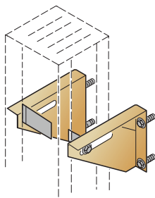
Рисунок 4-13 Крепежный кронштейн
