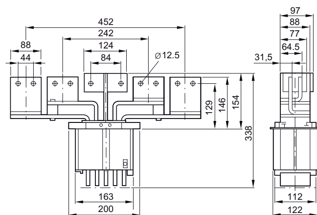
Рисунок 3-32 BD2.-1250-VE
