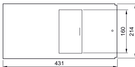
Рисунок 3-57 BD2-AK03M2/A...
