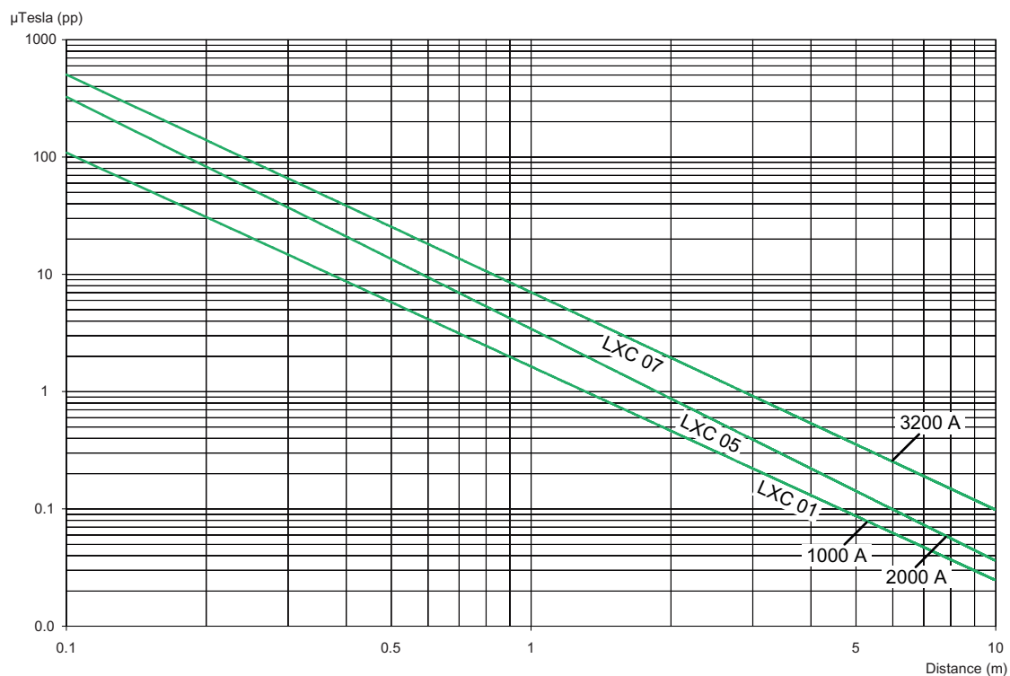
Рисунок 7-16 LXC магнитные поля для систем 1000 A, 2000 A и 3200 A
