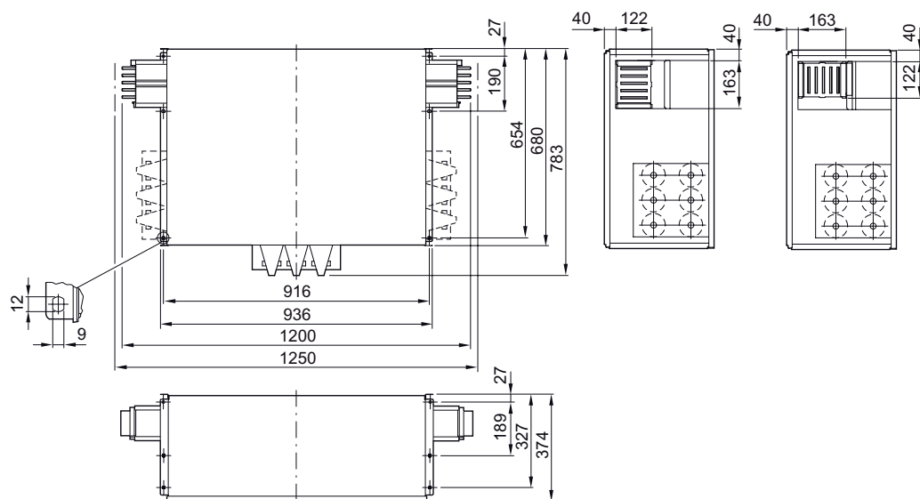
Рисунок 3-44 BD2.-1000-ME
