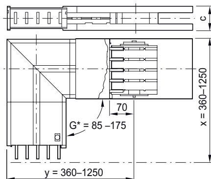
Рисунок 3-21 BD2.-....-LR-...(-G*), BD2.-....-LL-...(-G*)
