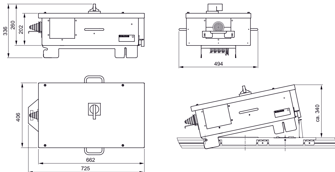
Рисунок 3-61 BD2-AK04/LSD...
