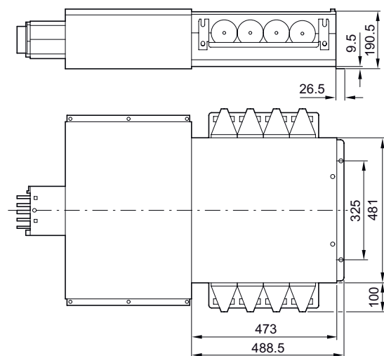
Рисунок 3-42 BD2-1250-KR (BD2.-1250-EE)
