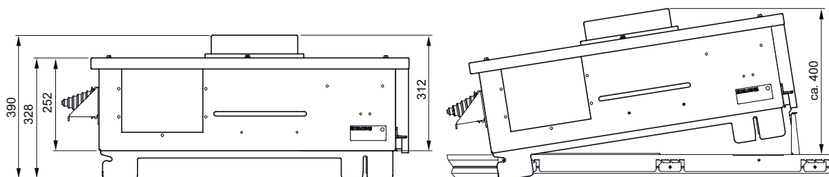
Рисунок 3-66 BD2-AK05/LSM..., BD2-AK06/LSM...
