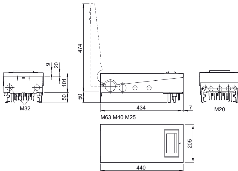
Рисунок 3-59 BD2-AK3X/GS00, BD2-AK3X/GB
