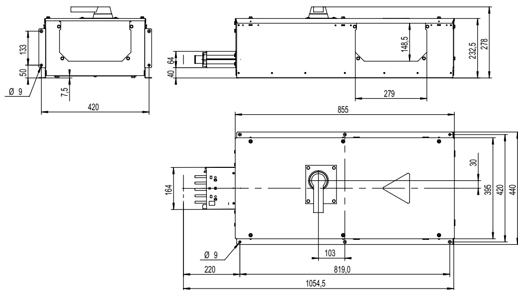
Рисунок 3-37 BD2C-250-EESC, BD2C-315-EESC
