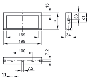
Рисунок 3-73 BD2-400-BB, BD2-1250-BB
