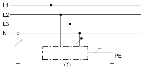
Рисунок 7-4 ТТ система
