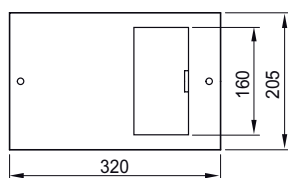
Рисунок 3-69 BD2-GKM2/F
