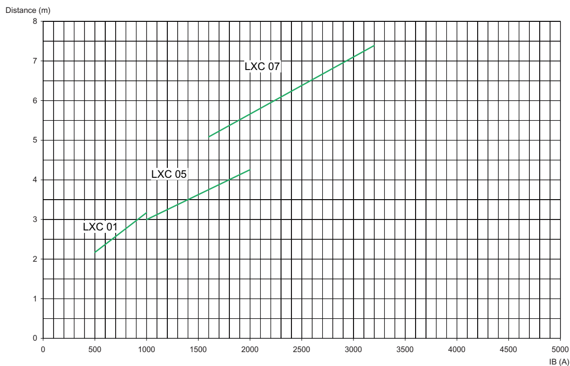
Рисунок 7-17 LXC профиль расстояния нагрузки для 0.2 \mu\text{T} системы 1000 A, 2000 A и 3200 A
