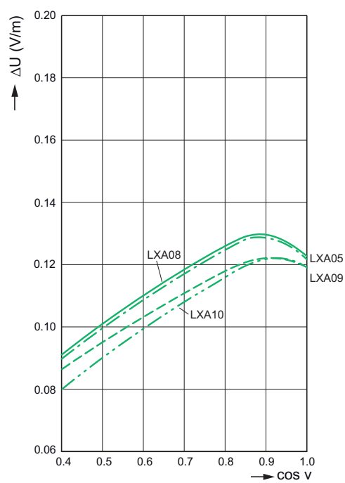
Падение напряжения LXA
