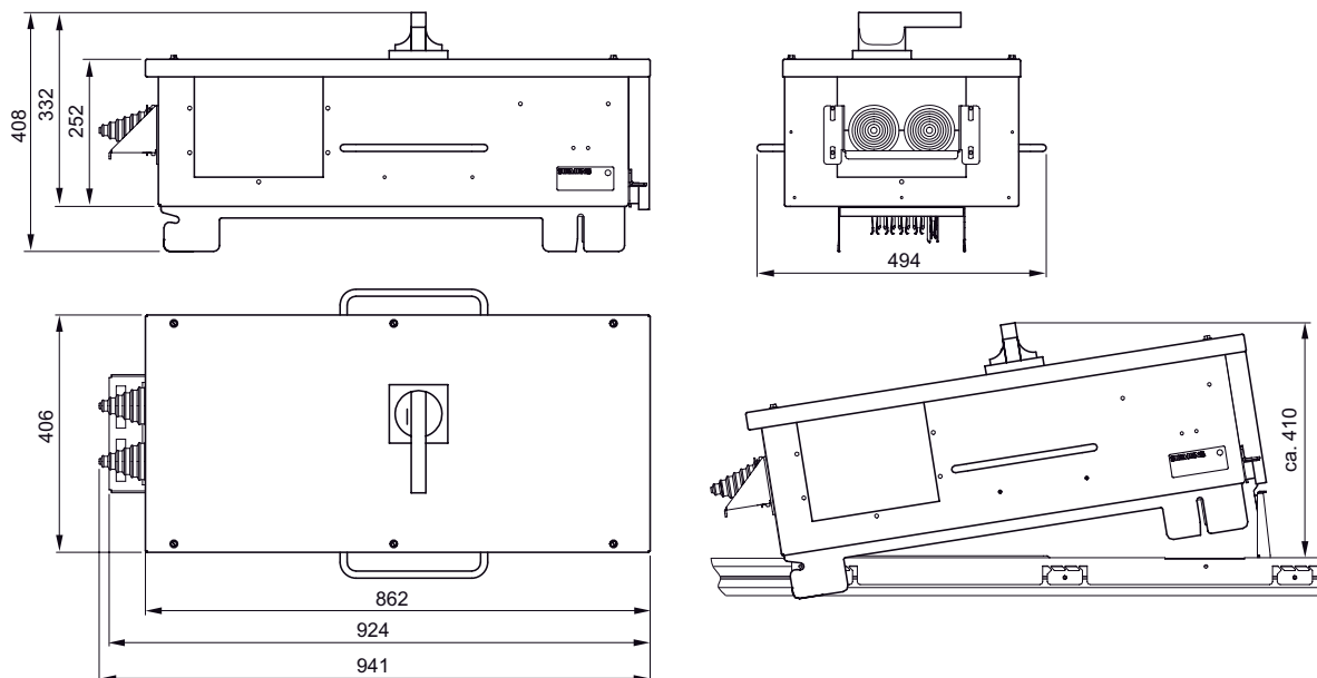
Рисунок 3-65 BD2-AK05/LSD..., BD2-AK06/LSD...
