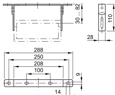
Рисунок 3-75 BD2-BD
