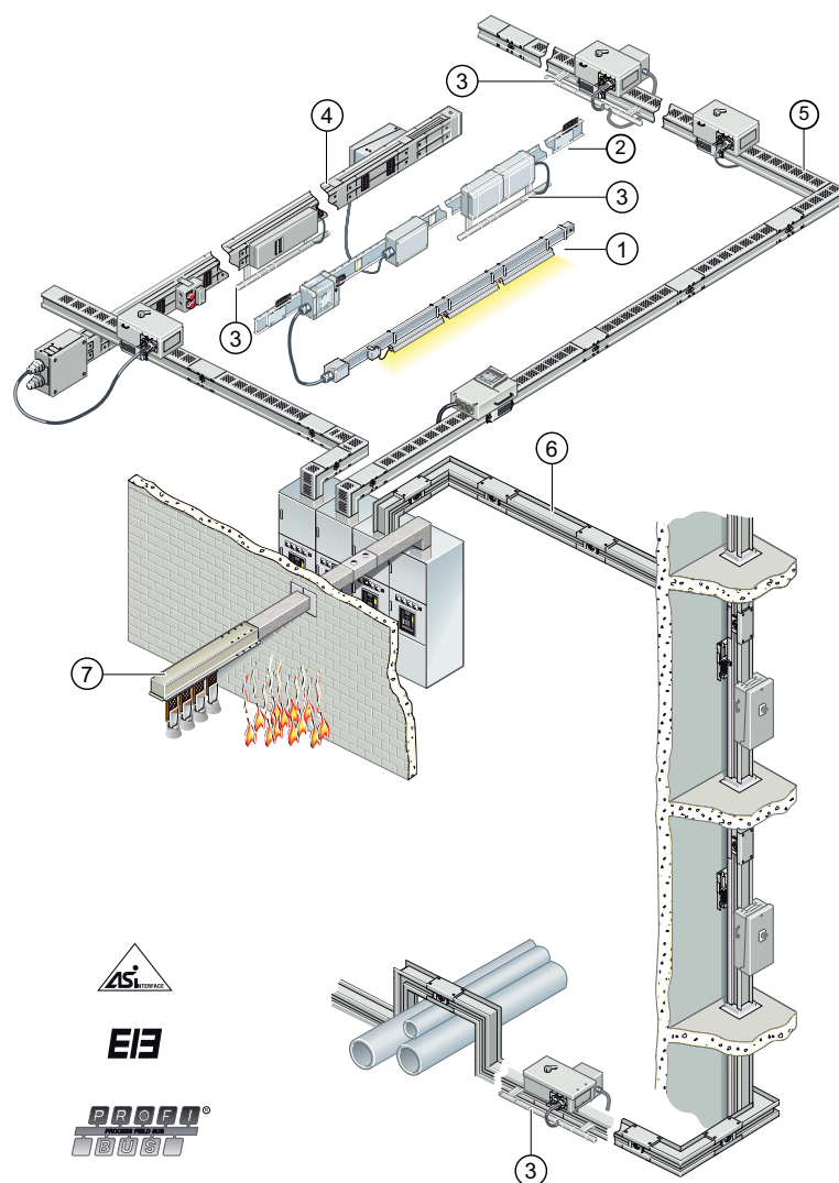
Рисунок 1-1 Обзор систем шинопроводов
