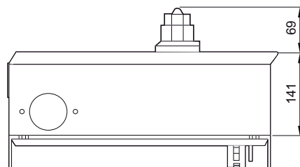
BD2-AK03X/FS...
