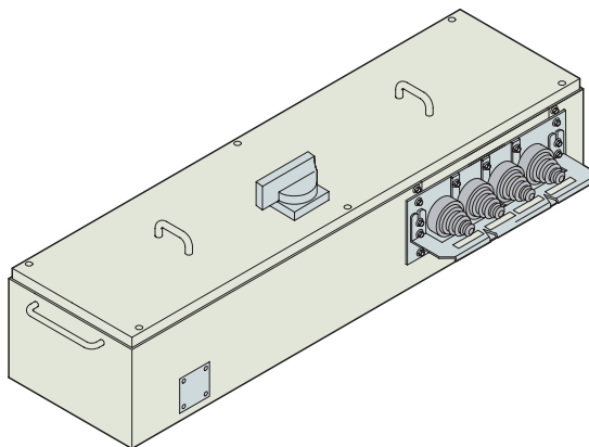
Рисунок 5-9 Предварительно устанавливаемые ответвительные коробки от 800 А до 1250 А
