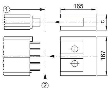
Рисунок 3-72 BD2-400-FE, BD2-1250-FE
