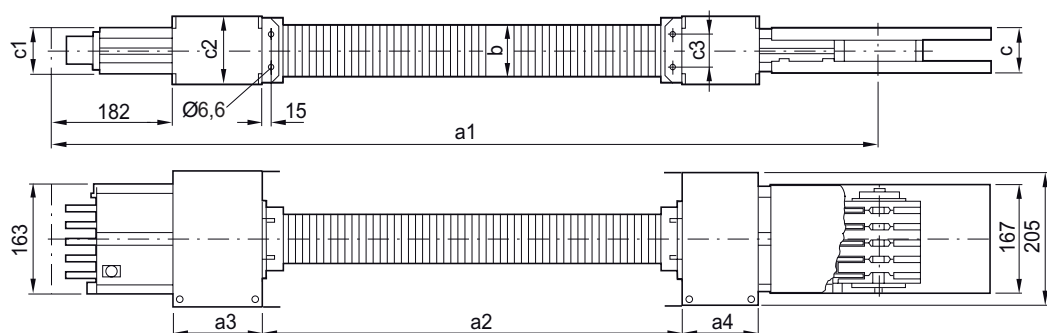
Рисунок 3-29 BD2-400-R, BD2-800-R
