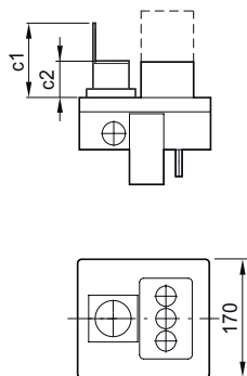
Рисунок 3-48 BD2-AK1/CEE165...
