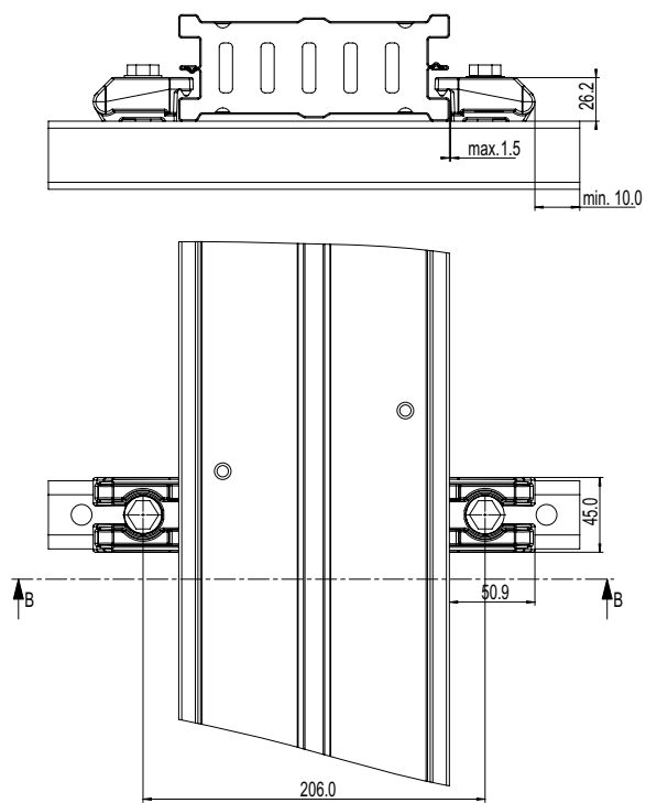
Рисунок 3-76 BD2-BVC
