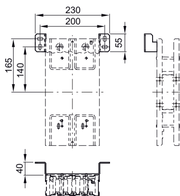
BD2-BVF
