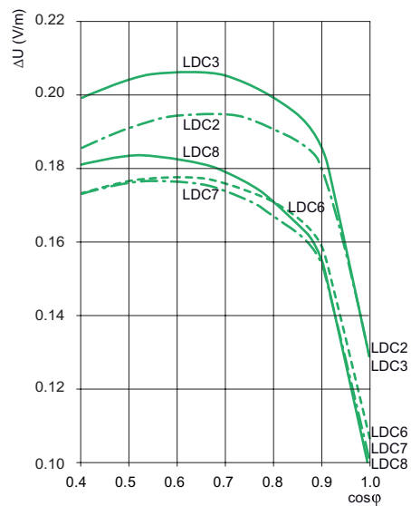
Падение напряжения LDC
