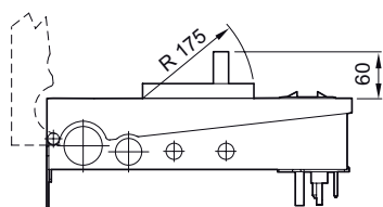
Рисунок 3-60 BD2-AK3X/GSTZ00
