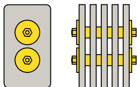
Рисунок 6-8 Стыковочный узел
