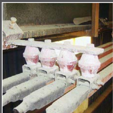
"Троллейные шинопроводы с защитой Dura Coat" на процессинговом кране электролитического производства, Чили
