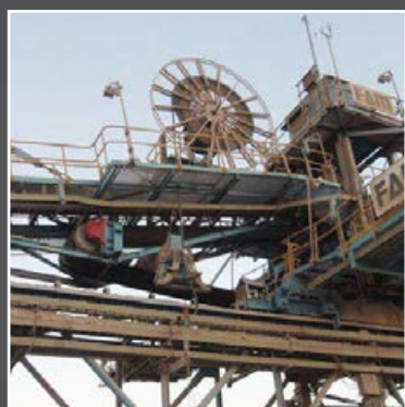
Приводной кабельный барабан на сбрасывателе, Чили
