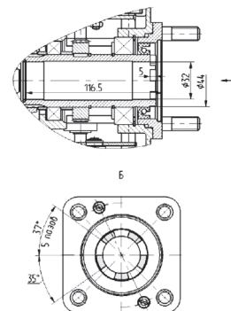
Механизм МЭМ2-100-01АП
