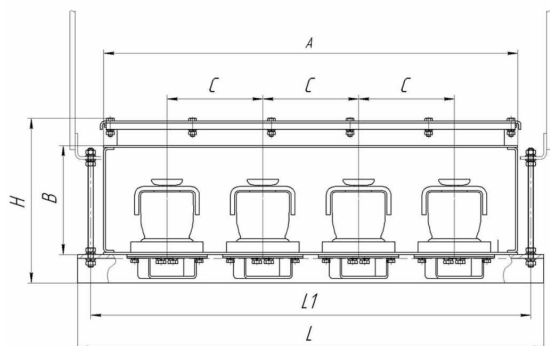
Токопроводы серии ТЗП на 0,4 кВ.
