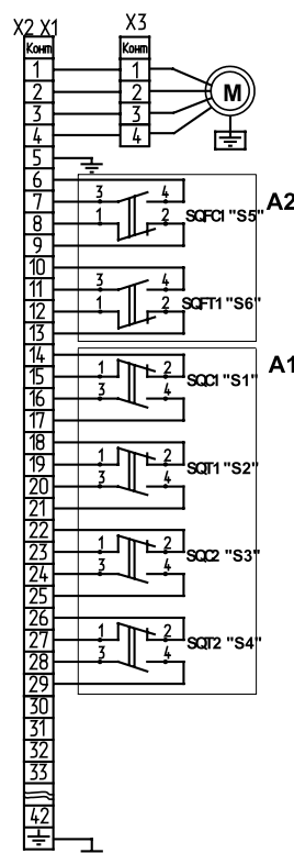
Рисунок С.3 – Схема электрическая принципиальная МЗО(Φ)-40-08КАМ с БКВ и ограничителем момента.
