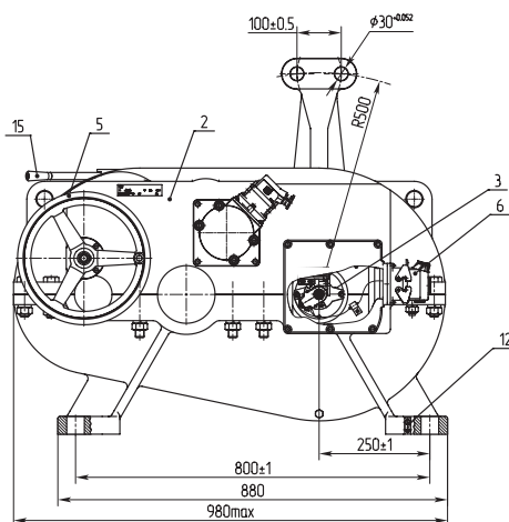
а) Механизм с разъемом "HARTING"
