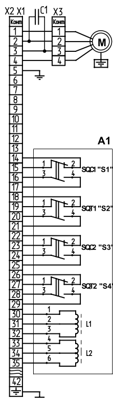
Рисунок С.5 – Схема электрическая принципиальная МЗО(Φ)-40-08А с БСПИ.
