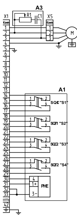
Рисунок С.10 – Схема электрическая принципиальная МЗО-250-08А с БСРТ.
