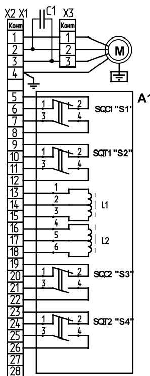
Рисунок С.6 – Схема электрическая принципиальная МЗО-40-01А, МЗО-40-93А с БСПИ.
