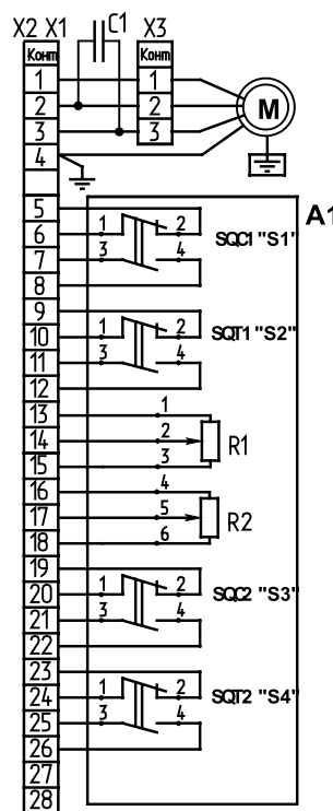
Рисунок С.3 – Схема электрическая принципиальная МЗО(Φ)-40-08КАМ с БКВ и ограничителем момента.
