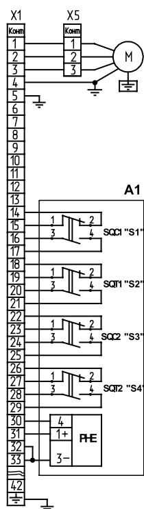
Рисунок С.9 – Схема электрическая принципиальная МЗО(Ф)-250-08КА с БСРТ.
