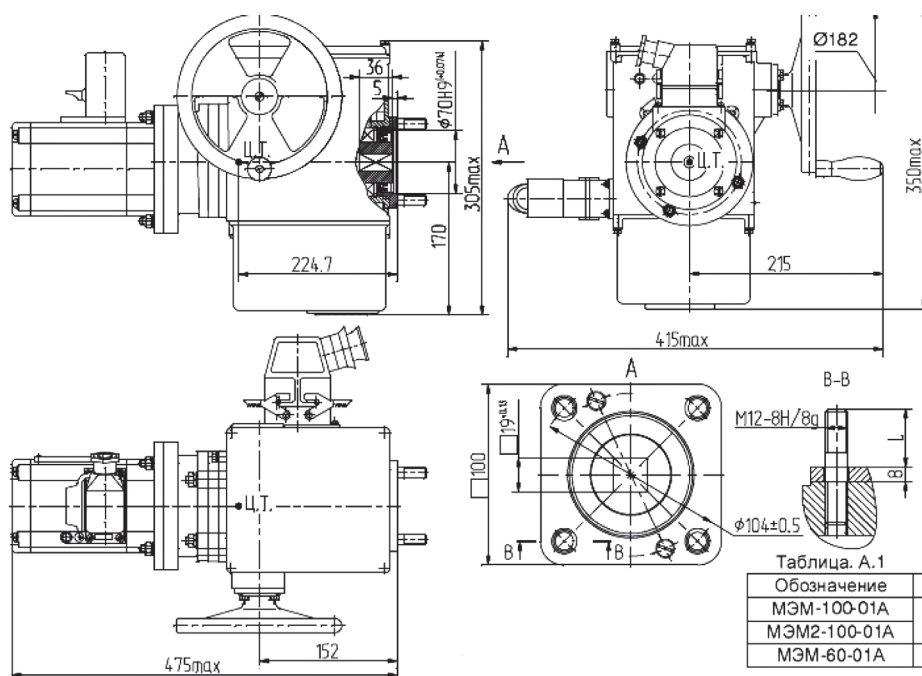
Механизмы МЭМ-100-01АO и МЭМ-100-01АП
