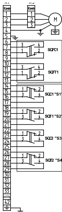
Рисунок С.12 – Схема электрическая принципиальная МЗО(Ф)-250-08КАМ с БКВ.
