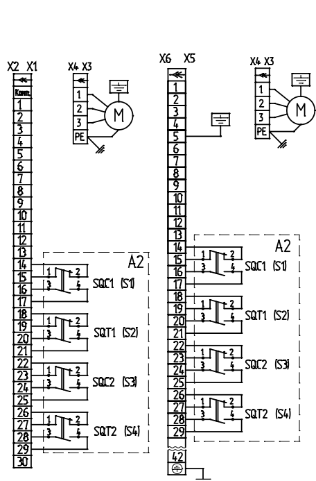
Рисунок С.32 – Схема электрическая принципиальная МЭОФ-4000-99КА.
