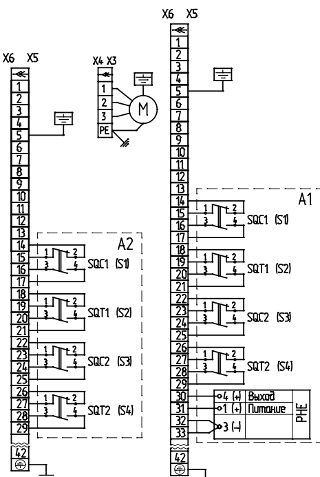
Рисунок С.33 – Схема электрическая принципиальная МЭОФ-4000-99КА с разъемом HARTING.
