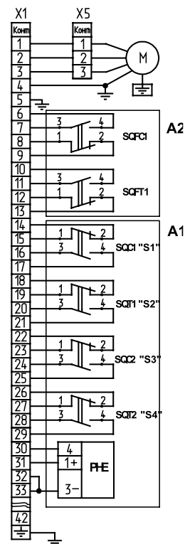
Рисунок С.11 – Схема электрическая принципиальная МЗО(Ф)-250-08КАМ с БСРТ с ограничителем момента.
