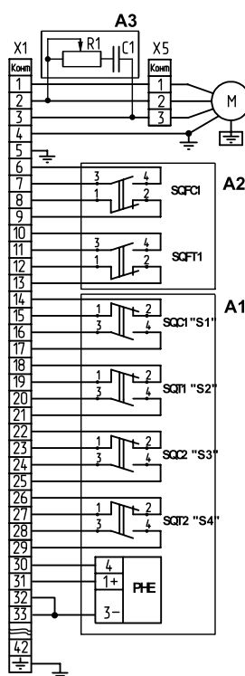
Рисунок С.13 – Схема электрическая принципиальная МЗО-250-08АМ с ограничителем момента и БСРТ.
