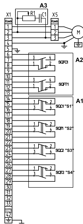
Рисунок С.14 – Схема электрическая принципиальная МЗО-250-08АМ с ограничителем момента и БКВ.
