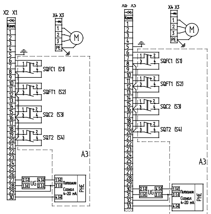
Механизм с разъемом РП10-30
