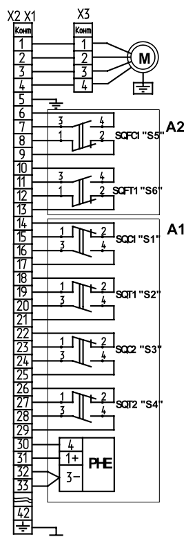
Рисунок С.2 – Схема электрическая принципиальная МЗО(Φ)-40-08КАМ с БСПТ и ограничителем момента.
