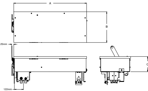
Рис. 2. Отводной блок на ток 252 - 500 A
