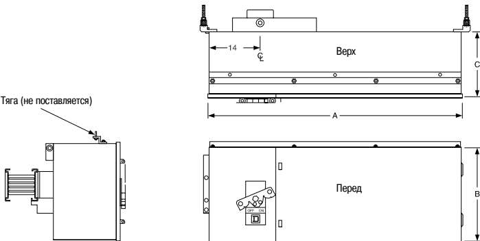
Рис. 3. Отводной блок на ток 630 - 1000 A
