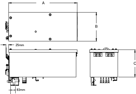
Рис. 1. Отводной блок на ток 16 - 250 A
