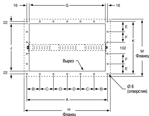
Размеры выреза и разметочный шаблон для фланца секции на ток от 630 до 6300 A
