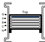
Внутренняя шина заземления
