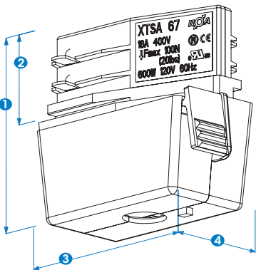
XTSA 67 1. 60 mm 2. 28 mm 3. 60 mm 4. 32 mm
