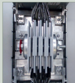
Самопозиционируемое кассетное соединение
