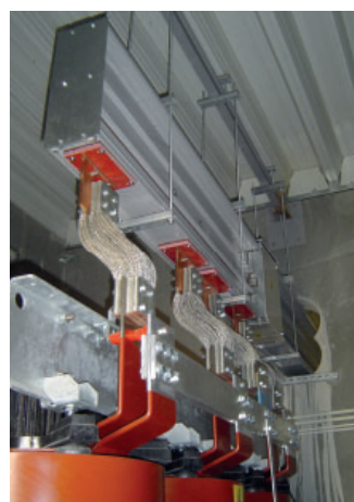
Подключение шинопровода к трансформатору (тип 1) гибкими конструкциями
