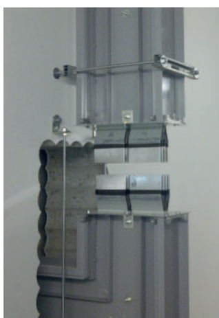
Шинопроводы Power Xpert® XP перед монтажом кассетного соединителя (фотография конструкции)
