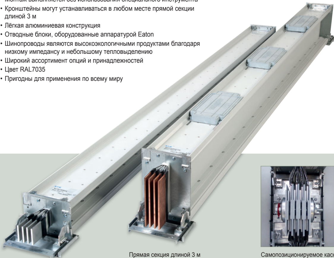
Прямая секция длиной 3 м
